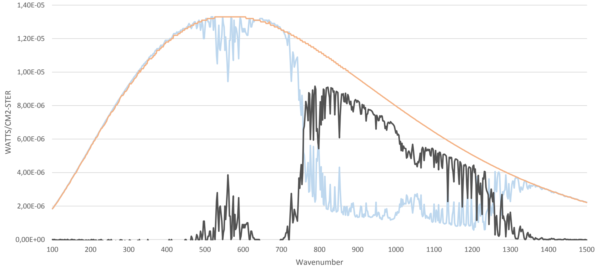
Modtran , Surface (US std atm, clear sky)
